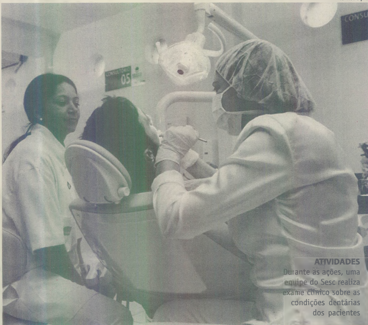
REPRODUÇÃO
