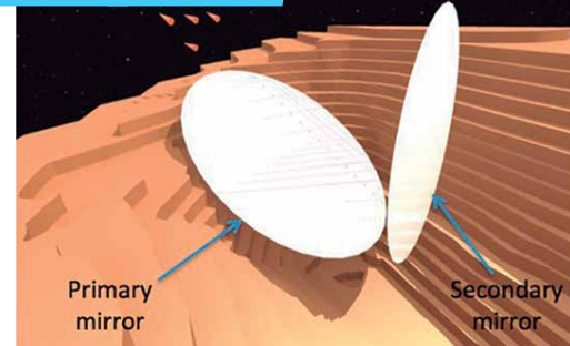
Imagem detalha o funcionamento do radiotelescópio que vai medir oscilações de matéria no universo
