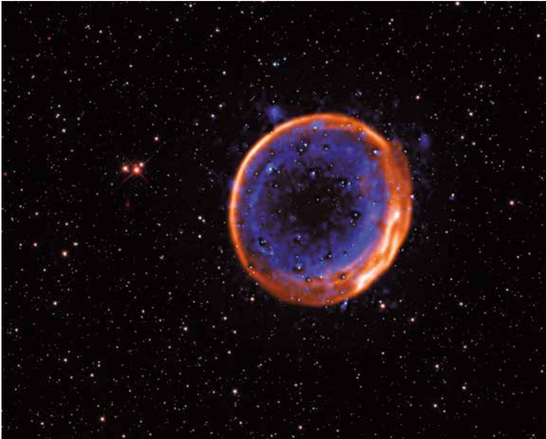
Imagem da supernova SNR 0509-67.5, que sofreu duas detonações capturada pelo Very Large Telescope
