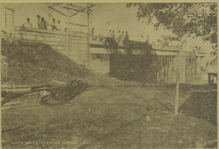
Ponte sobre o rio Santo Antonio, entre Assú e Mossoró, Rio Grande do Norte.
