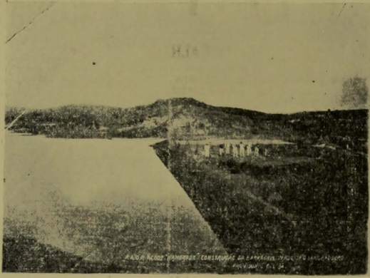
Acude "Namorado", em S. João do Cariri, que está sendo construído pelo Estado em cooperação com a Inspetoria de Obras Contra as Secas.
