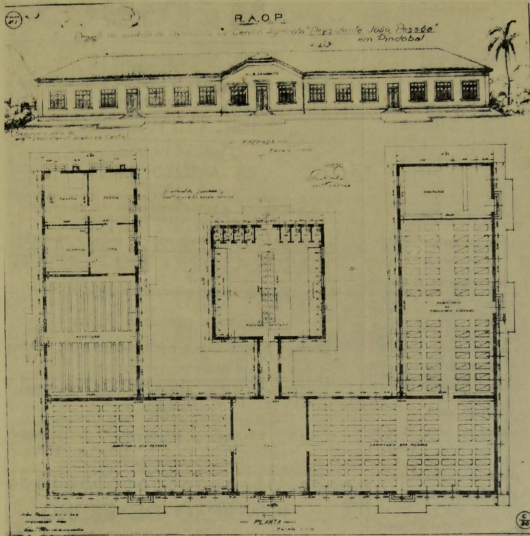
Projeto do pavilhão de alojamento em construção no Centro Agrícola "Presidente João Pessoa", em Pindobal.
