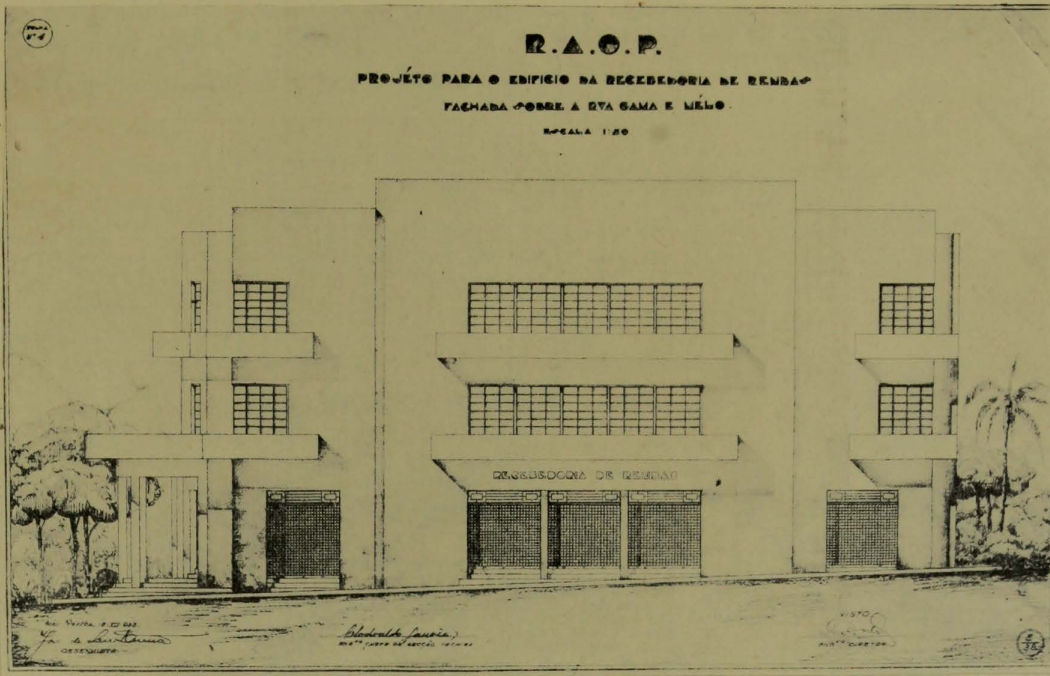
Planta da edificio da Recebedoria de Rendas, em construção à praça Arruda Camara.
