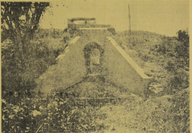
ESTRADA JOAO PESSOA-SANTA RITA — Um dos boeiros construidos pela Directoria de Obras Publicas.
