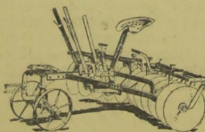
Cultivador "John Deere" 5 enxadas n. 8 — com alavanca.
