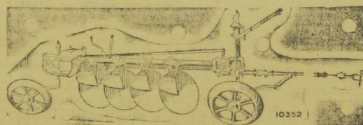
rollamentos esfericos proprio para o tractor Twenty-Two. Arado especial "RANSOMES" de 4 discos, equipado com
