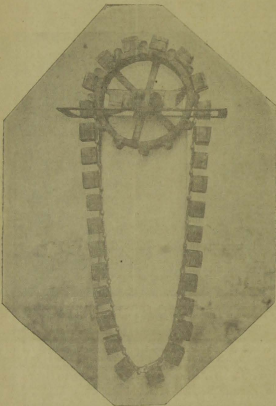
A nora em miniatura, construída para experiencia, mostrando alguns dos seus detalhes
