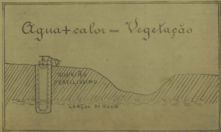
A nora será verdadeiramente ideal se obedecerem, na montagem, ás indicações deste croquis
