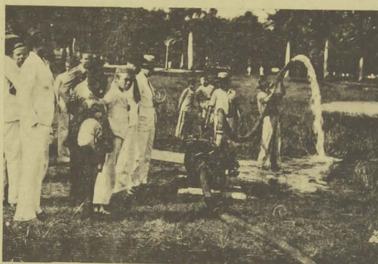
Um motor-bomba arranca do sub-solo a agua que inutilmente corre lá e leva-a ás plantas sedentas, nas grandes estiadas. Si os fazendeiros da região sertaneja possessem dessas machinas não precisariam viver sobressaltados pela dolorosa expectativa de um anno máo. A Direcçõria de Produccão pode fazer experiencias, nos municipios de Pianó, Cabaceiras, Picuhy, Catolé do Rocha e Souza, na propria terra do lavrador interessado.
