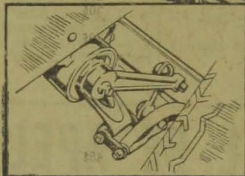
Amortecedores ajustaveis, de dupla accão, para controle das 4 rodas.
