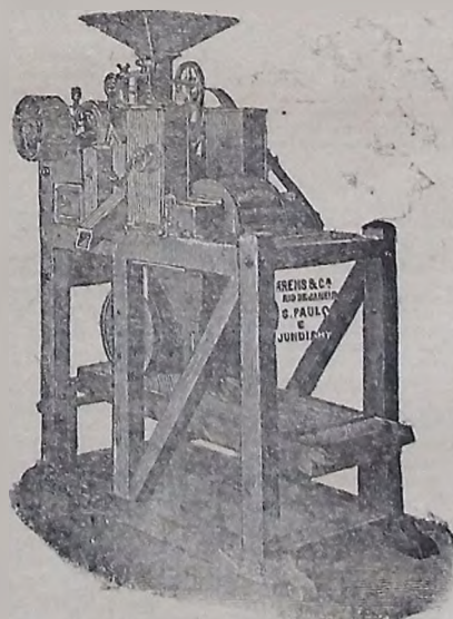
MACHINA PARA BENEFICIAR ARROZ PAULISTA
