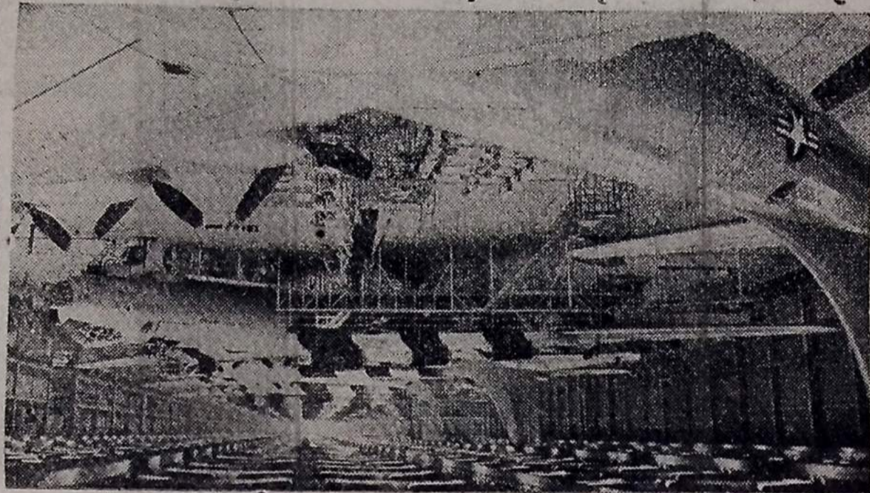
Uma linha de montagem dos B-36, o grande bombardeiro que é o maior avião da força aérea dos Estados Unidos. Com quasi 70 metros de envergadura de asas, o B-36 move-se diagonalmente ao longo da oficina que tem 60 metros de largura. Estes gigantes aviões são construídos pela Consolidated Vultee Aircraft Corp., em Fort Worth, Texas. (USIS)
