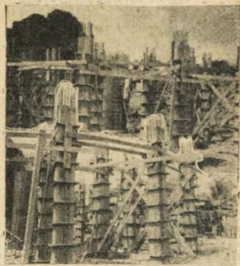
ENCONTRAM-SE em fase adiantada os trabalhos de construção de um reservatório d'água, com capacidade de 2.000 m 3 , na Rua Diogo Velho, e que se destina à distribuição da água vinda das adutoras de Marés. As fotos acima fixam um aspecto das obras de construção do referido reservatório, cuja conclusão se espera para breve.
