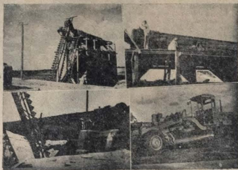
Os flagrantes acima foram tomados no acampamento da "Construtora Estevam Marinho", no local onde se concentra o maquinário pesado da Empresa. Vem-se, ao alto, à esquerda, o grupo formado pela Central de Britagem e Central de Concreto; ao lado, um detalhe da britadora. Em baixo, à esquerda, vista parcial da peneira vibratória e do elevador de caçambas; à direita, a moto-nivelador "Adams".
