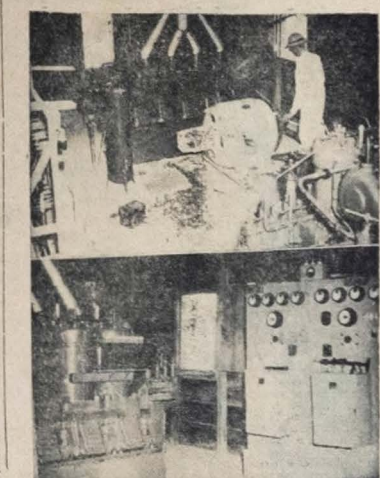
A CASA DE FORÇA — Dois flagrantes de Casa de Força, vendendo os dois potentes conjuntos eletrogênicos ao alto, e em baixo, o quadro sincronizador.
