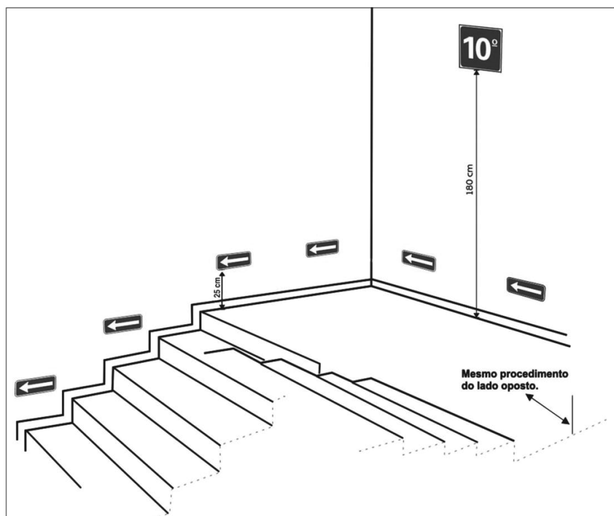
Figura C-8: Sinalização complementar. Exemplo de rodapé
