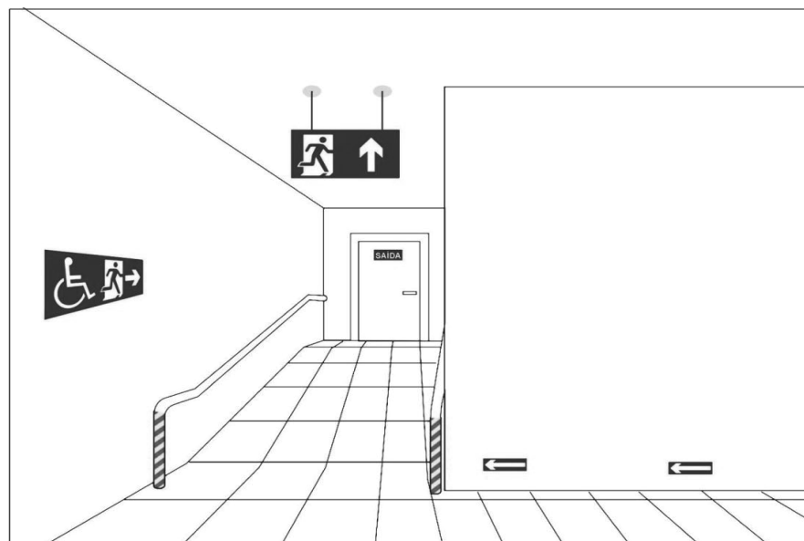
Figura C-15: Sinalização de saída em rampa.
