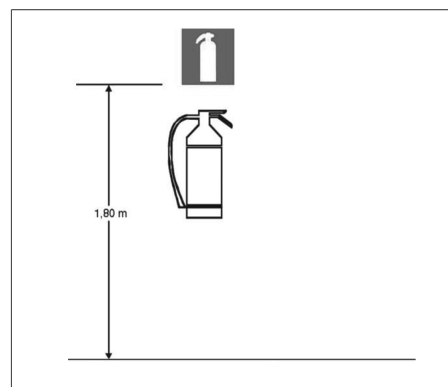
Figura C-6: Sinalização de extintores
