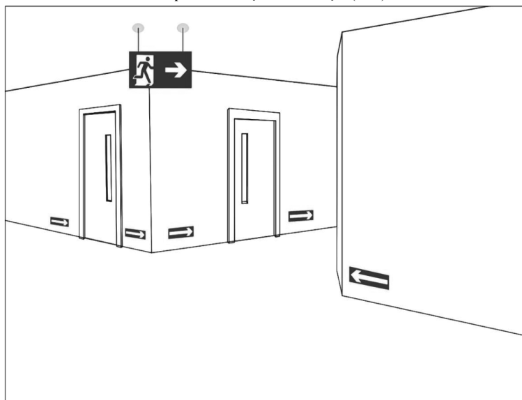
Figura C-13: Sinalização de saída perpendicular ao sentido da fuga, em dupla face.
