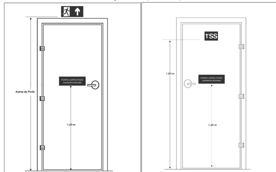
Figura C-1: Sinalização de porta corta-fogo (vista do hall)
