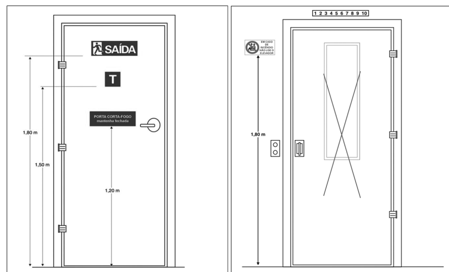
Figura C-3: Sinalização de porta corta-fogo (vista da escada)
